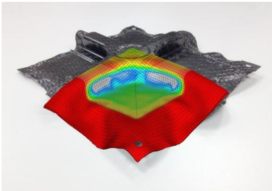
計算された温度分布を示す成形プロセスのシミュレーション（赤：220 °C, 青：210 °C） （写真：ランクセス AG）
